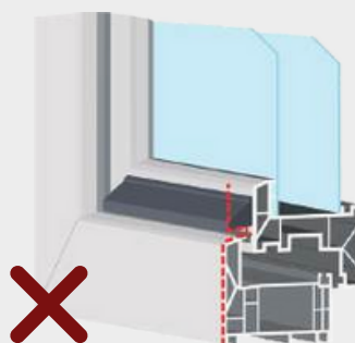
Ramy z profilem pogodowym
